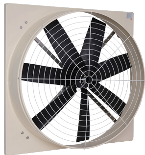
仕様 54インチ7枚羽根のDC簡易ファン 54インチ7枚羽根のDC換気ファン 54インチ3枚羽根のサーボ換気ファン
